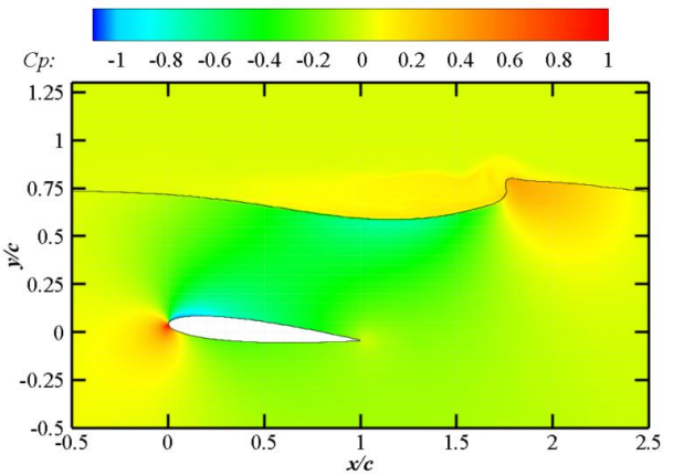
(D) h/c = 0.78
