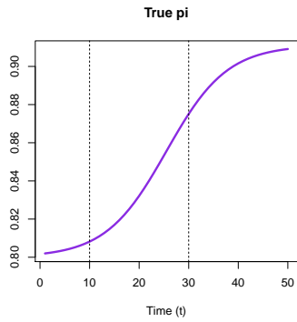
(g) True \pi(t) .
