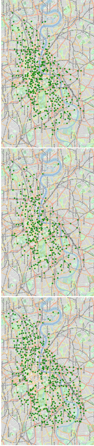
(a) Cluster D2 - 7 am.
