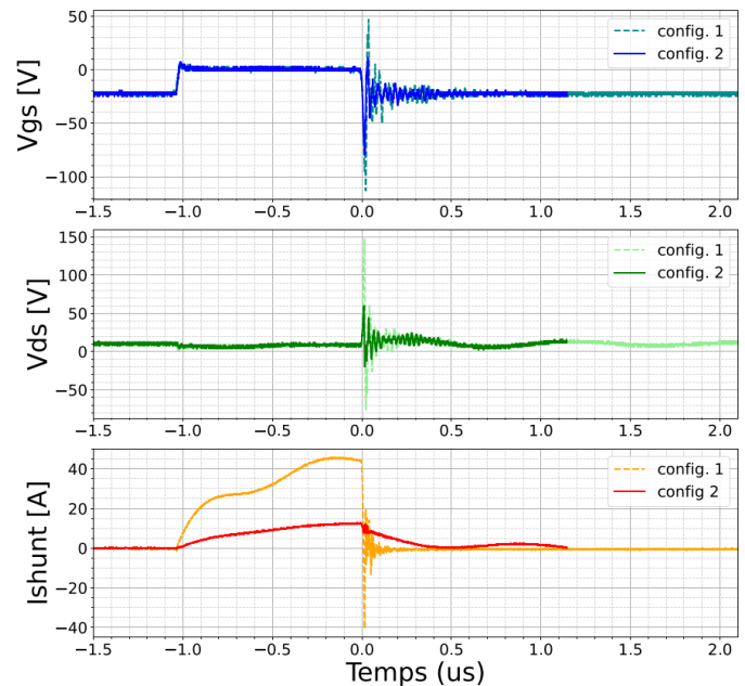
Figure 9 : essai en court-circuit pour V_{DS}=10 V (configurations 1 et 2)
