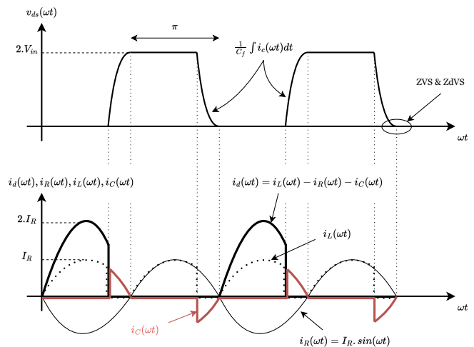
FIG. 3. Formes d'ondes théoriques obtenues avec un rapport cyclique inférieur à 50 % sur la commande du transistor
