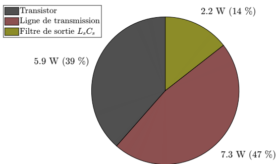
FIG. 15. Répartition des pertes dans le convertisseur d'après le modèle numérique pour V_{in}=28 V
