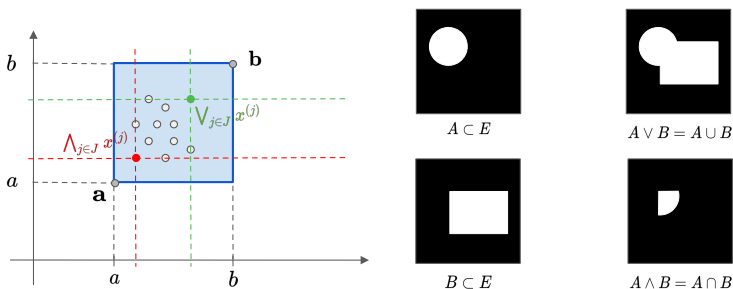
FIGURE 3.3 – Illustration des treillis complets de l'exemple 2 : [a, b]^n et \mathcal{P}(E) .
