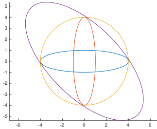
FIGURE 3.4 – Illustration de l'absence de supremum pour deux ellipses, montrant que (\mathcal{S}_n, \preceq) n'est pas un treillis complet, comme expliqué dans l'exemple 2.
