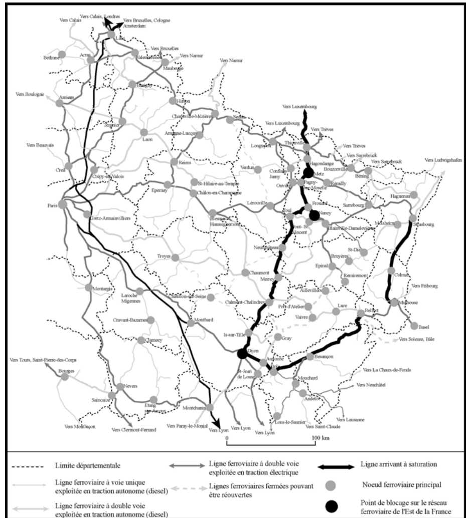
Figure 3 : Les points de blocage du réseau ferroviaire du Nord-Est de la France
