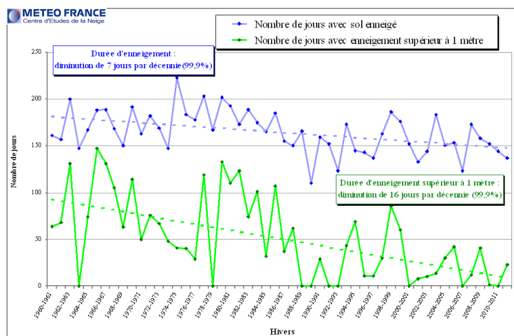
FIGURE 17 – Durée d’enneigement au col de Porte (1325 m, massif de Chartreuse). Source : http://www.cnrm-game.fr/IMG/pdf/lesaffaire_aic_2012.pdf
