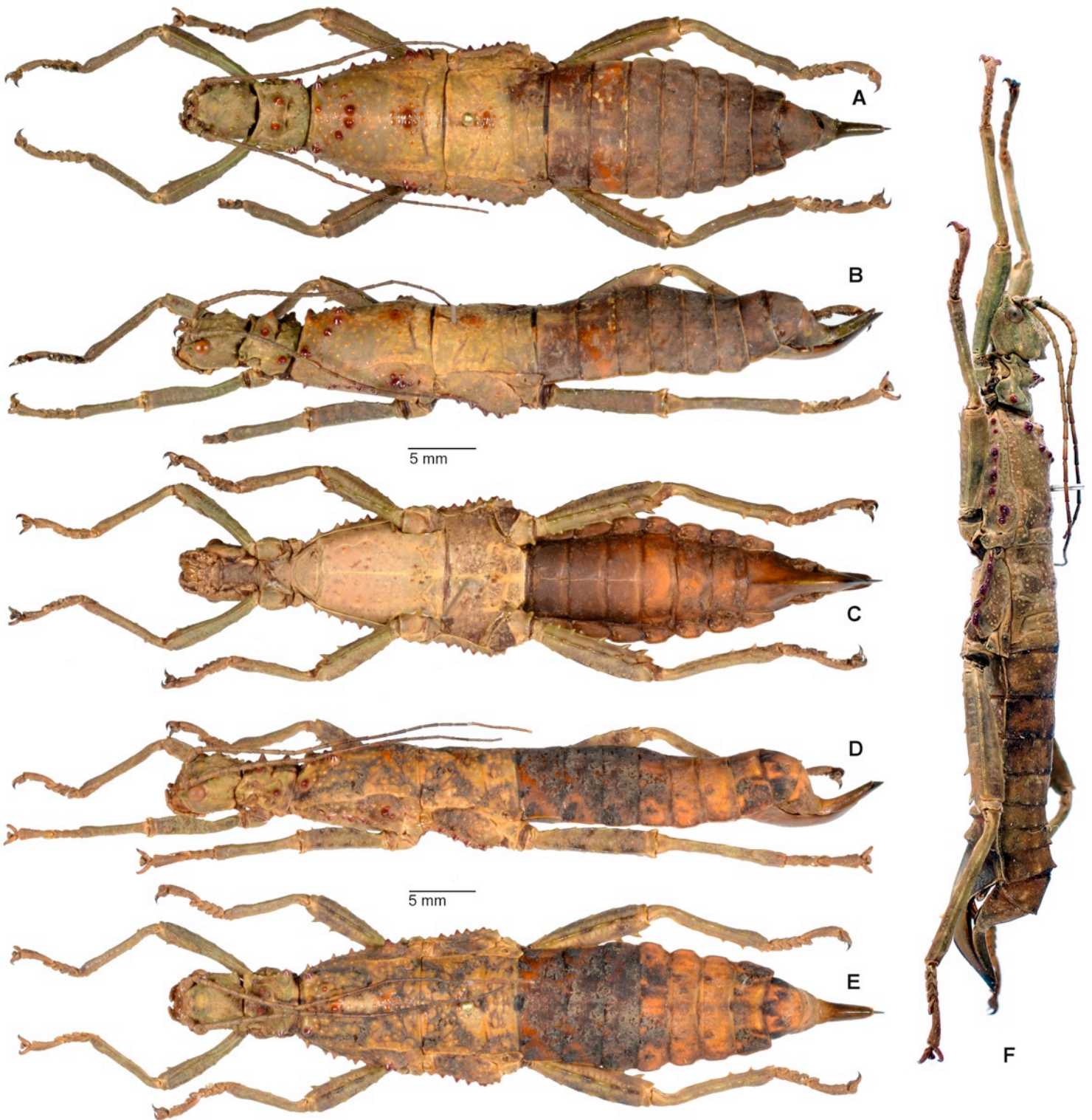
Fig. 1. Theramenes letiranti n. sp., ♀.
