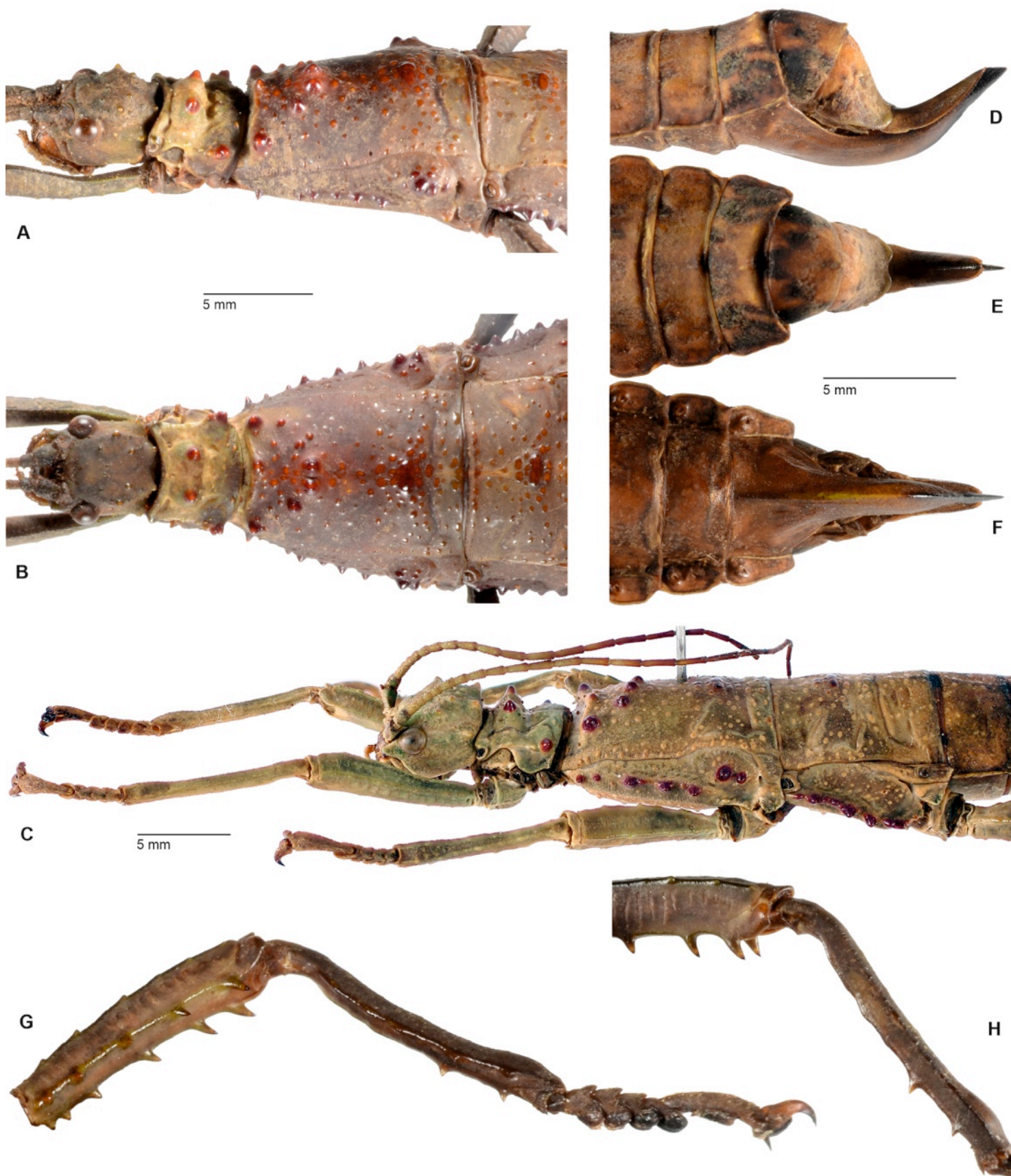
Fig. 2. Theramenes letiranti n. sp., ♀.
