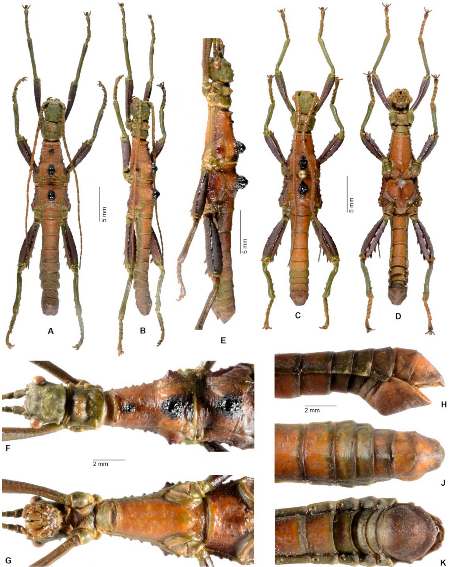
Fig. 3. Theramenes letiranti n. sp., ♂.
