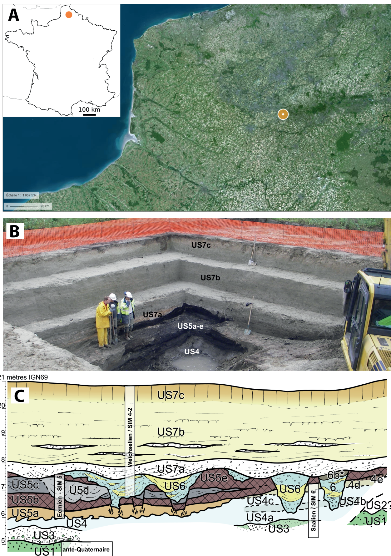
Fig. 1 : Présentation du site du Waziers.
