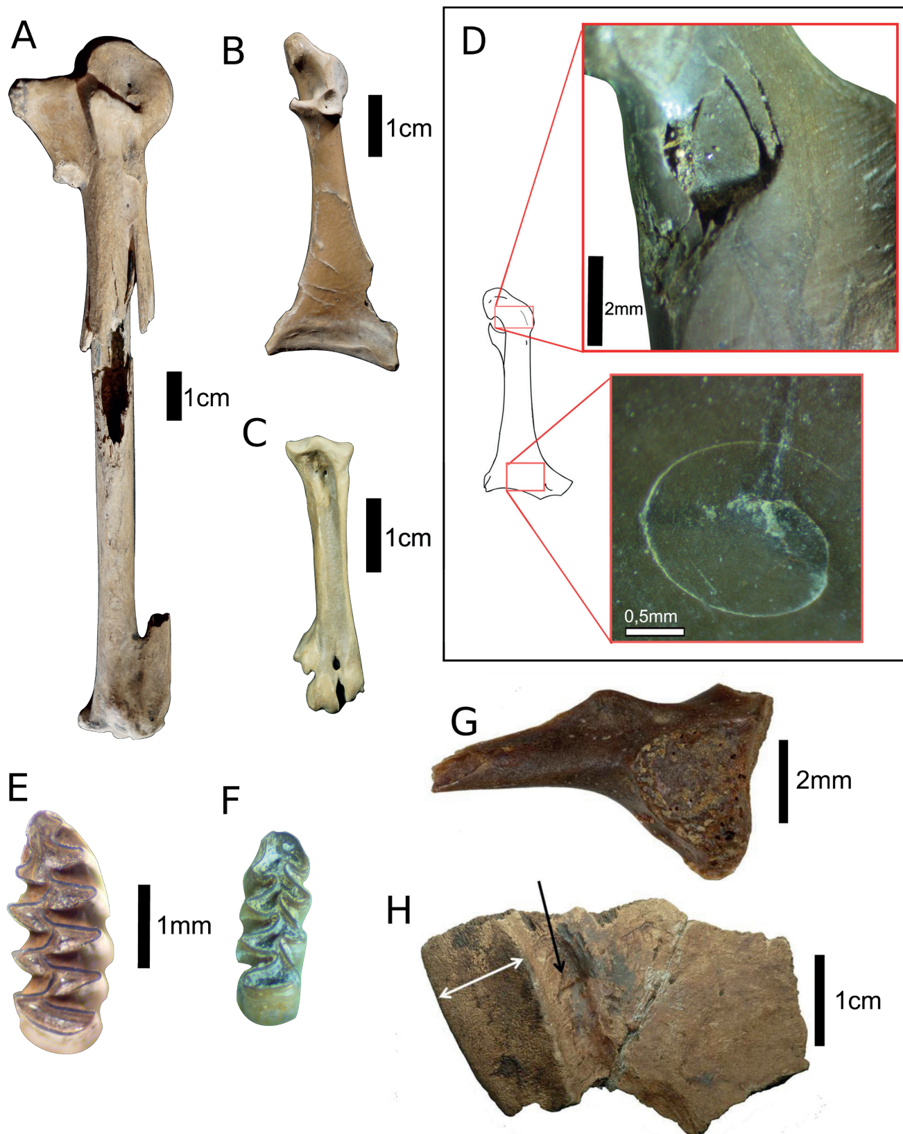
Fig. 2: Photographies de différents restes de petits vertébrés présents sur le site de Waziers.
