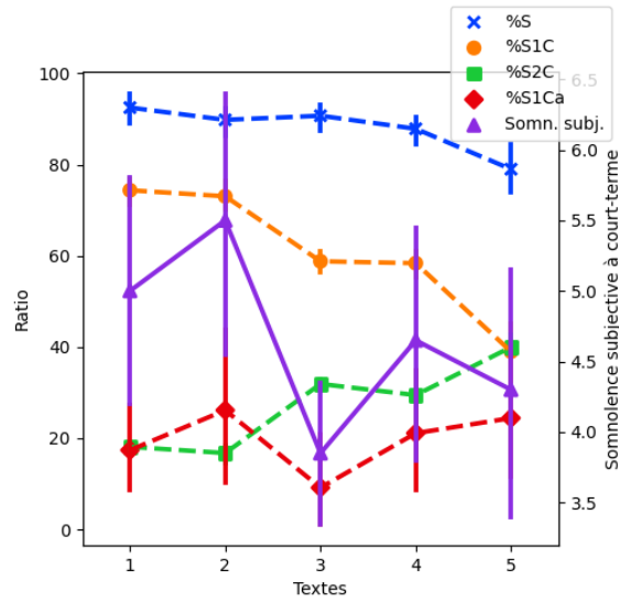
Figure 1. Variations intra-locuteur de la somnolence subjective à court-terme et des descripteurs ayant un effet significatif d'après l'ANOVA.
