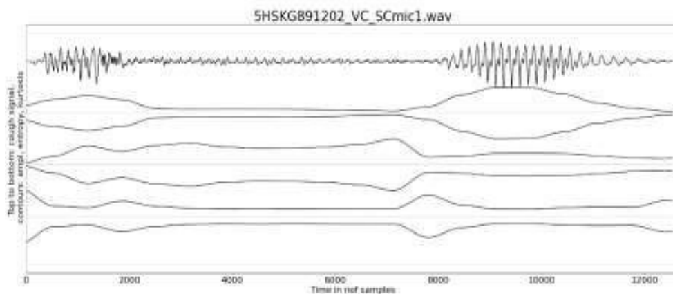
Figure 1. Une émission de toux volontaire d'un sujet sain ; première ligne (en haut) : le signal de toux original ; deuxième ligne : le contour d'amplitude ; troisième ligne : le contour d'entropie échantillonnée ; quatrième ligne : le contour de kurtosis
