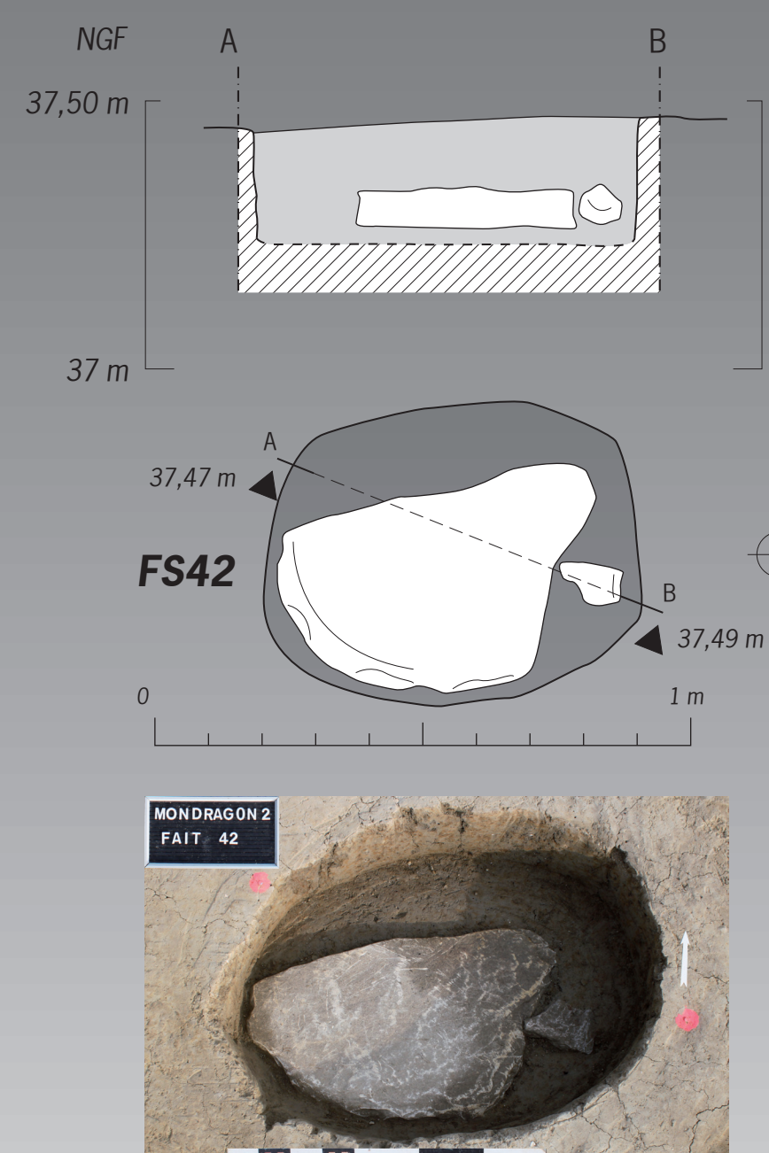
Dalle pour obturer le silos FS42 (Rel. et DAO N. Bourgaire)
