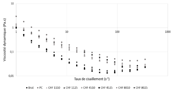
Figure 2 : Analyses rhéologiques
