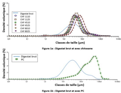
Figure 1 : Analyses granulométriques
