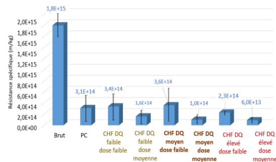
Figure 2 : Résistances spécifiques à la filtration
