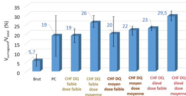
Figure 1 : Performances de décantation
