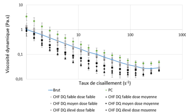
Figure 3 : Comportement à l'écoulement
