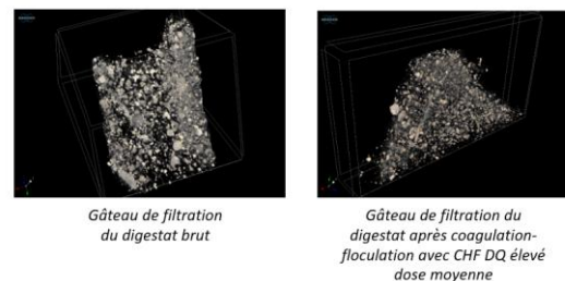
Figure 4 : Images par microtomographie
