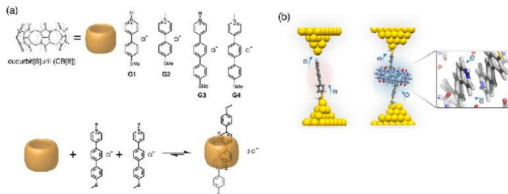
Figure : (a) Représentation schématique des structures moléculaires utilisées pour étudier le transport de charge intermoléculaire faisant intervenir la dimérisation dans des macrocycles cucurbiturils ; (b) Représentation schématique des jonctions moléculaires formées par une molécule unique de pyridinium et un complexe hôte-invité d'un dimère. Extrait du Journal of the American Chemical Society 154, 6132 (2022). Copyright 2022 American Chemical Society.
