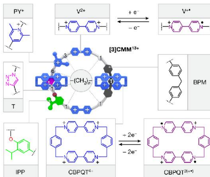
Figure : Moteur moléculaire basé sur un [3]-caténane combinant des anneaux de cyclobis(paraquat-p-phenylene) CBPQT4+, des unités viologène V2+, pyridinium PY+, triazole T, isopropylphénylène IPP et bis(4-méthylène-phényl)méthane BPM. Bleu : état redox oxydé, violet : état réduit. Springer Nature.
