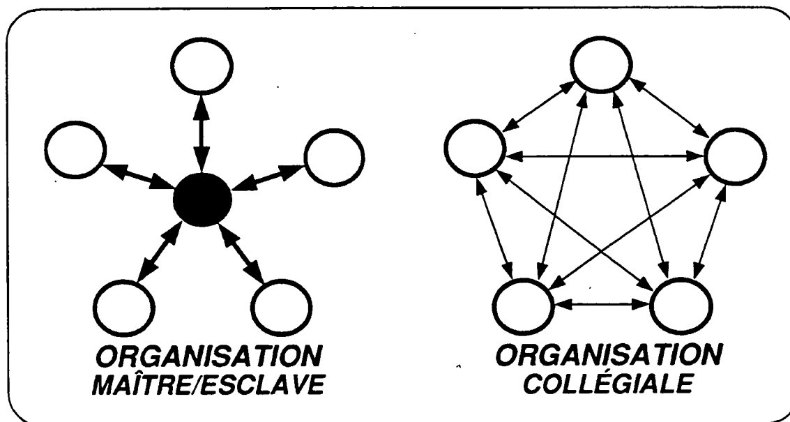
Figure 1. Schémas de communication typiques pour deux organisations fonctionnelles de processeurs en parallèle
