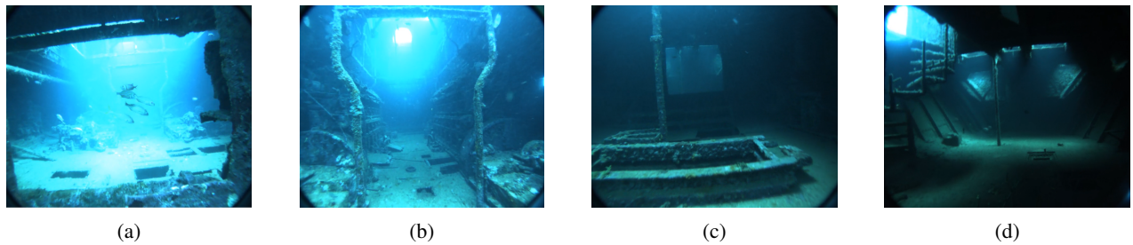
Fig. 4: A/In dataset [1]
