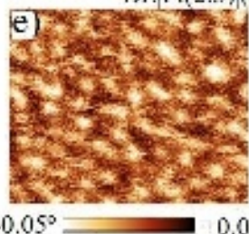
Bi 1 |Pt(2.3)|(Pt(5)|Co(1.6)|Ru(1.4)) 20
