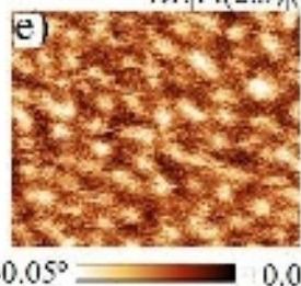
Bi|Pt(2.3)|(Pt(5)|Co(1.6)|Ru(1.4)) 20
