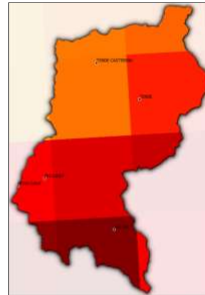
Tx07 2081-2100 RCP 8.5
