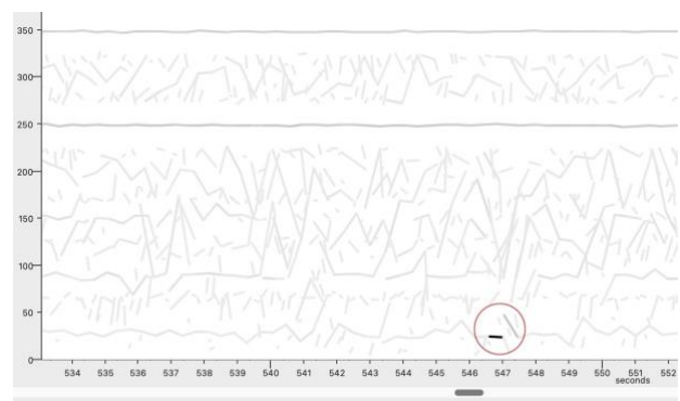
Figure 6. Analyse FFT du signal du mycélium au moyen du logiciel SPEAR, recherche de singularités (entourée en rouge).
