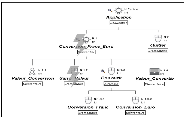
Figure 1 : Modèle de tâches K-MADe du Convertisseur.
