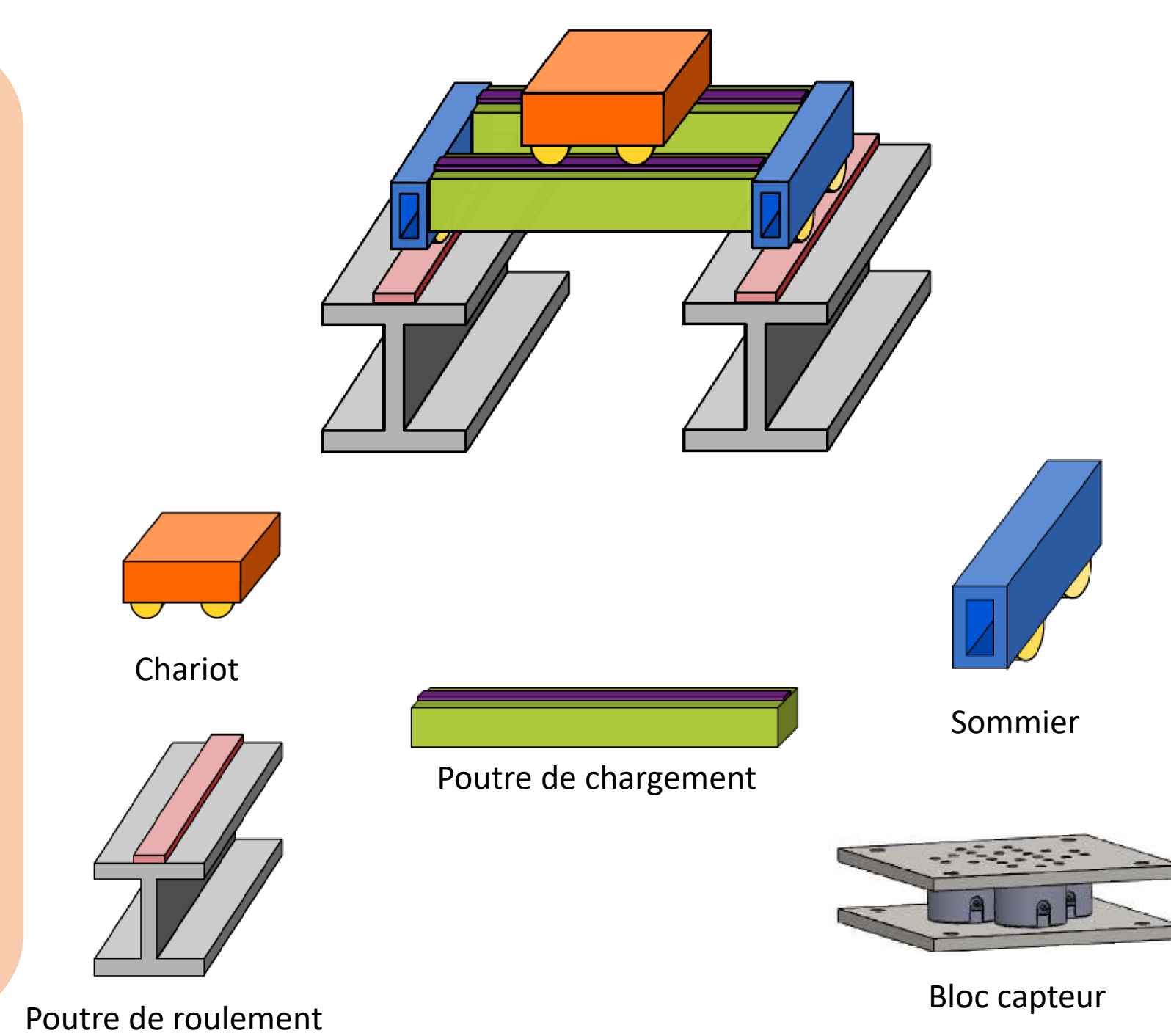
Campagne d'essais réalisée en 2015 sur la Table vibrante AZALEE (Laboratoire EMSI CEA, Saclay) dans le cadre d'une action collaborative entre l'IRSN, le CEA et EDF.
