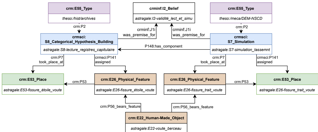
FIGURE 3 – Diagramme de mapping pour la mise en donnée d'un résultat de simulation prenant pour prémisses une hypothèse issue d'une source archivistique (CRMcore, CRMsci, CRMinf)
