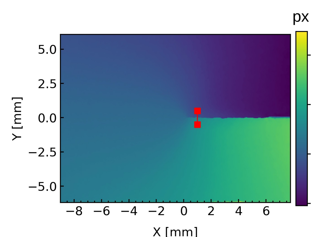
Jauge de mesure du COD sur le champ des déplacements à 1mm de la pointe
