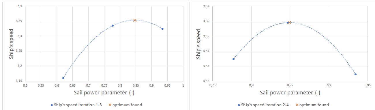
(a) Sail power parameter optimisation using points 1-3 (b) Sail power parameter optimisation using points 2-4
