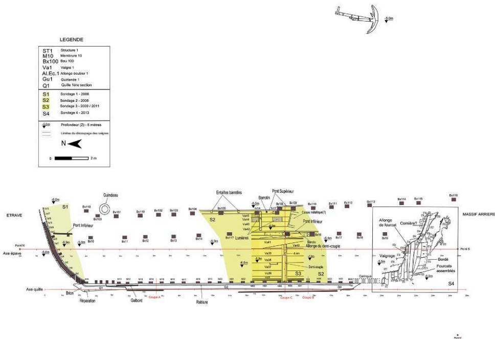
Fig. 1 – Planimétrie générale
