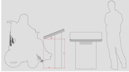
Fig. 2. Dimensionnement de la borne Autonomade
