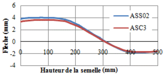
Figure 14 : Flèche semelle de poteau raidie et non raidie
