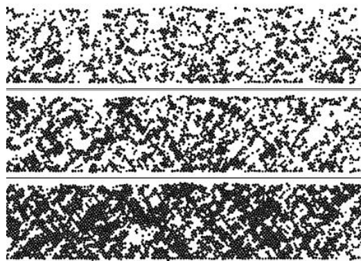
FIG. 7 – Distribution spatiale des grains surcontraints (en noir) pour \theta = 0 , \theta = 10 et \theta = \theta_c (de haut en bas).
