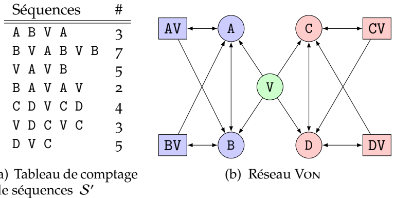
FIGURE 2 – Exemple d’utilisation des réseaux d’ordre séquentiel supérieur pour le clustering . Dans les séquences S' (tableau 2a), en passant par V en venant de \{A, B\} ou \{C, D\} , il est uniquement possible de retourner dans le même ensemble. Le réseau VON (figure 2b) contient deux composantes fortement connexes pouvant être retrouvées avec un algorithme de partitionnement de graphe (couleurs des nœuds). L’état V est ainsi présent dans les deux groupes.
