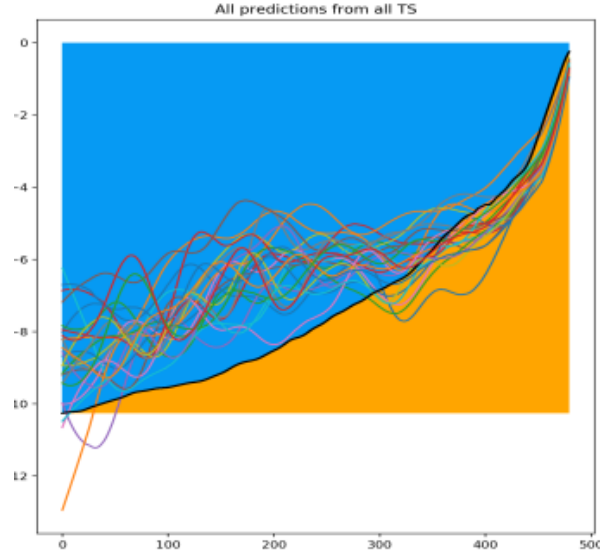
FIGURE 3.9 – Estimation de profils de plage par réseaux de neurones - cas réaliste (plage Gran Popo, Bénin) : prédictions de la bathymétrie à différentes dates et pour différentes conditions de vagues (courbes de couleur) vs profil moyen. Figure tirée de Benschila et al. (2020) [7]
