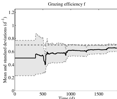
FIGURE 2.3 – Evolution temporelle de la moyenne (courbe noire) et de la moyenne plus/moins un écart type (zone grise) des paramètres estimés. Elles correspondent aux moyennes de ces quantités calculées sur 20 expériences. La valeur "vraie" correspond à la courbe noire pointillée. Figure tirée de Simon et Bertino (2012) [127].
