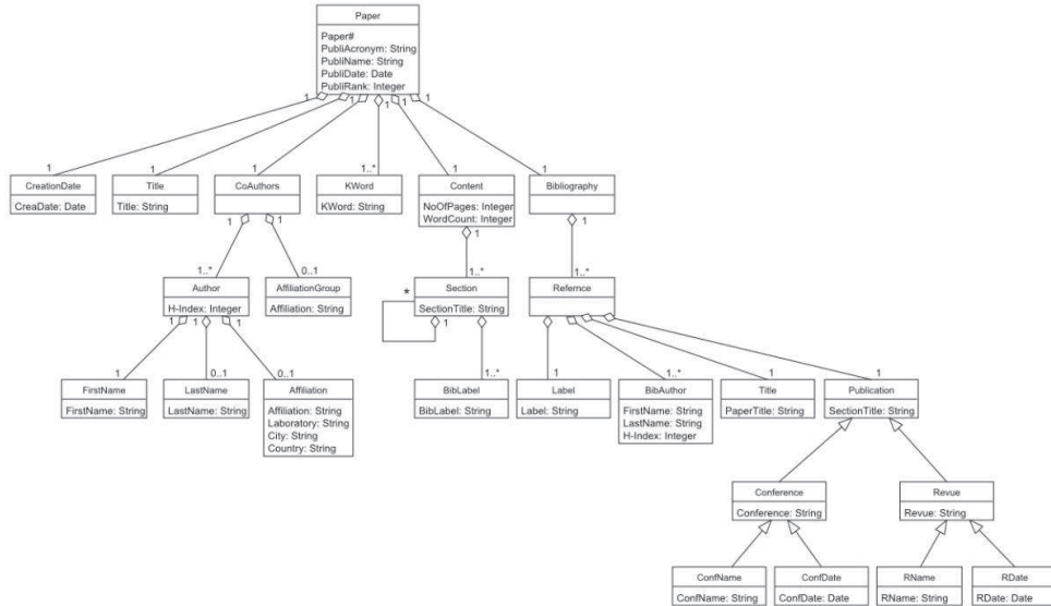
FIG. 4 – SourceCD représentant une classe de documents d'articles scientifiques.
