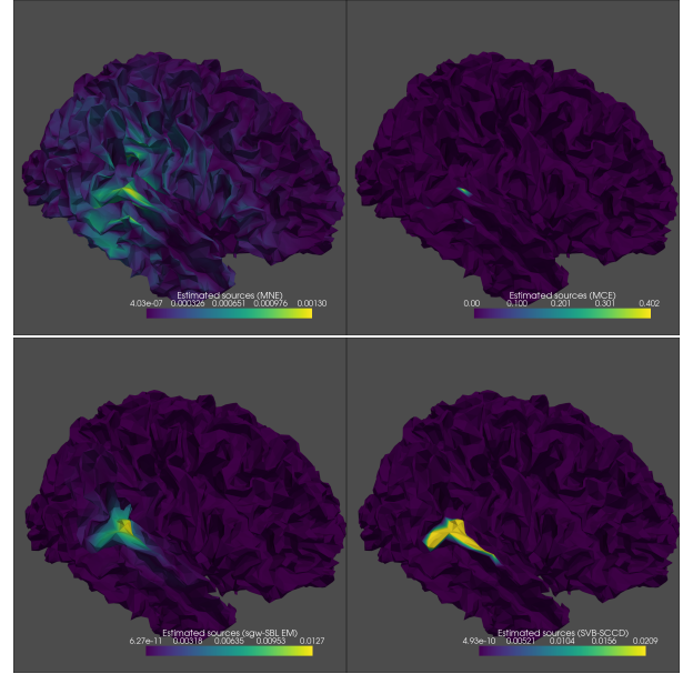
FIGURE 1 : Potentiels évoqués auditifs : cartes d'amplitude (8) pour les solutions MNE (haut gauche), MCE (haut droite), sgw-SBL EM (bas gauche) et SVB-SCCD (bas droite).
