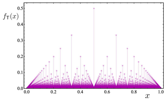
FIG. 2. Thomae function (15).
