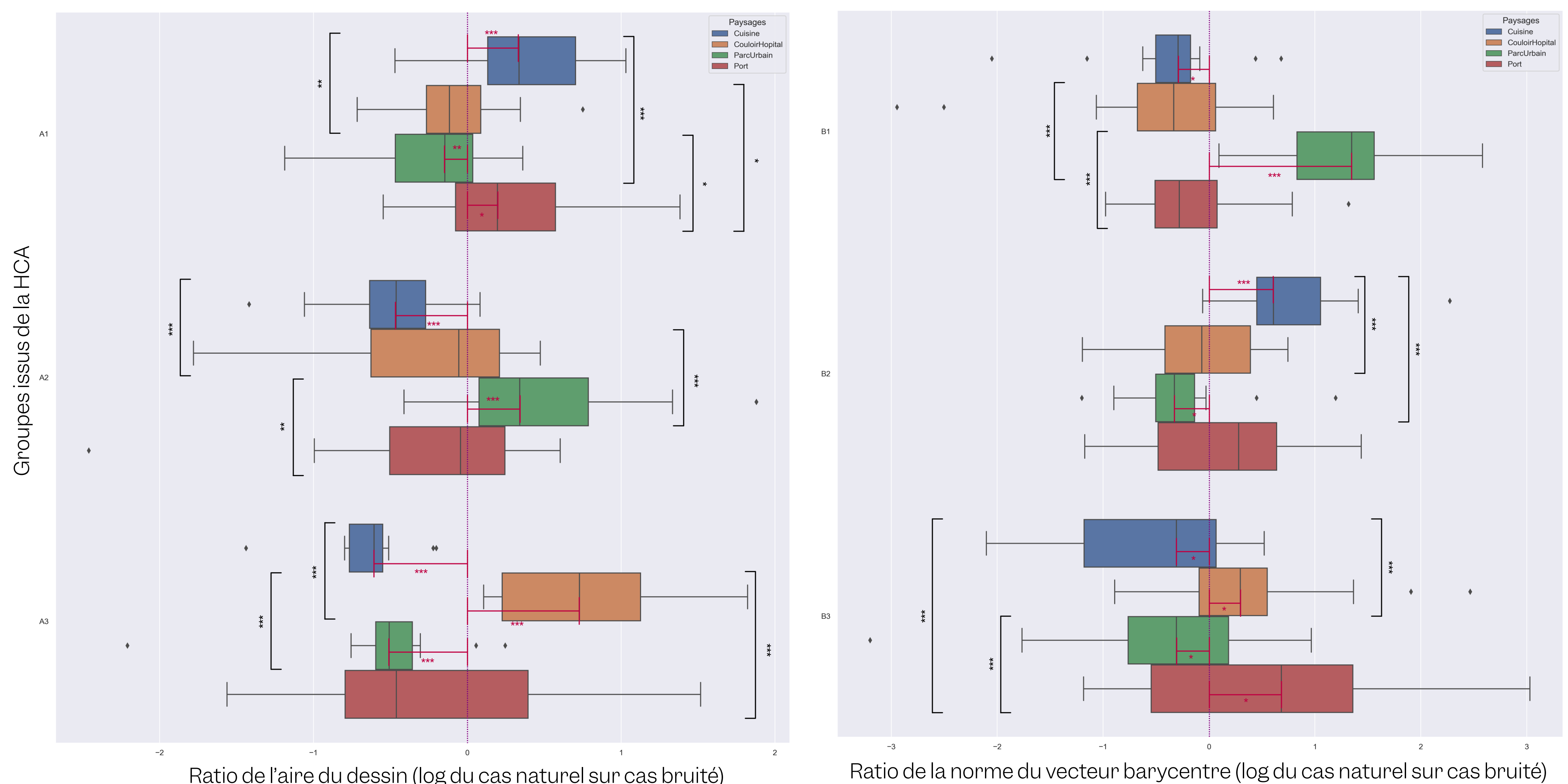
Boîtes à moustaches des résultats pour deux des variables analysées : l'aire du dessin et la norme du vecteur. Tout ce qui est au dessus de 0 veut dire que la variable observée est supérieure dans le cas naturel par rapport au bruité et en dessous, l'inverse. ***: p < 0.001 , **: p < 0.01 , *: p < 0.05 pour paysages, ***: p < 0.001 , **: p < 0.01 , *: p < 0.05 pour le contexte
