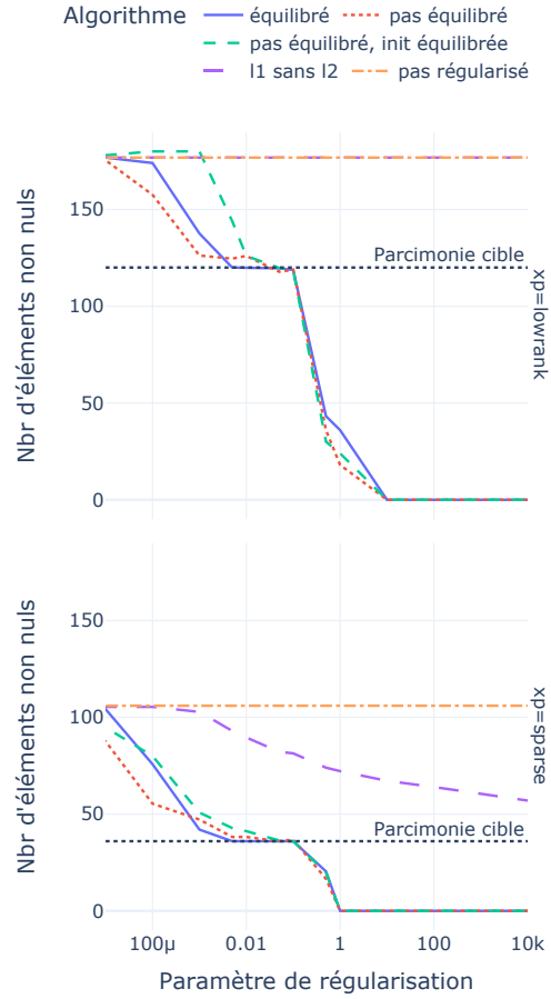
FIGURE 1 : Parcimonie du premier facteur en fonction du paramètre de régularisation \mu .
