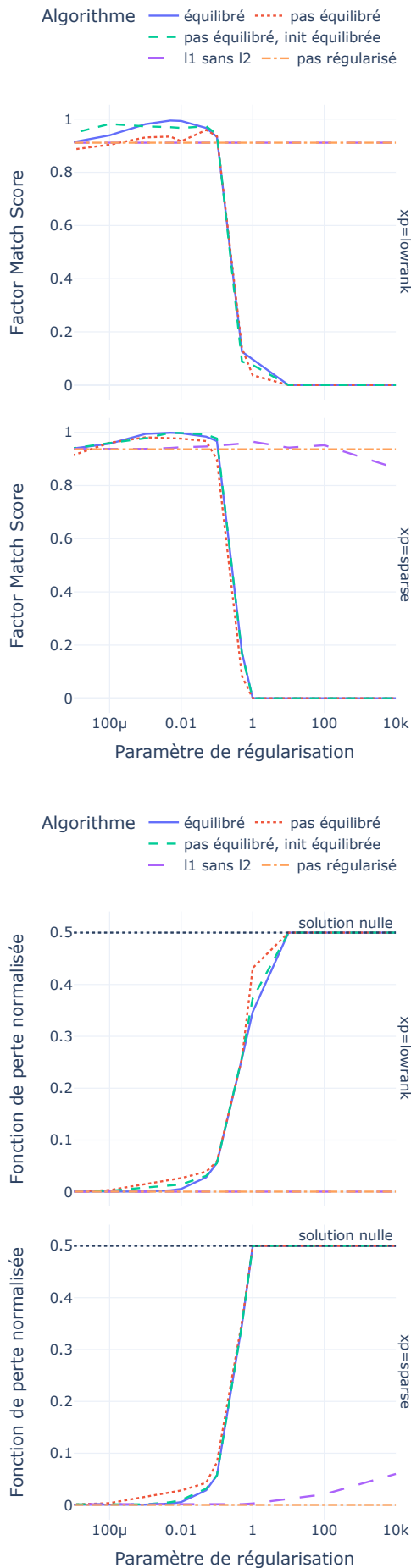
FIGURE 2 : (haut) FMS et (bas) fonction de perte en fonction du paramètre de régularisation \mu .
