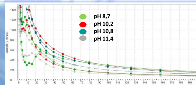
Viscosité des barbotines en fonction du pH
