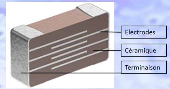
Schéma en coupe d'un condensateur multicouche
