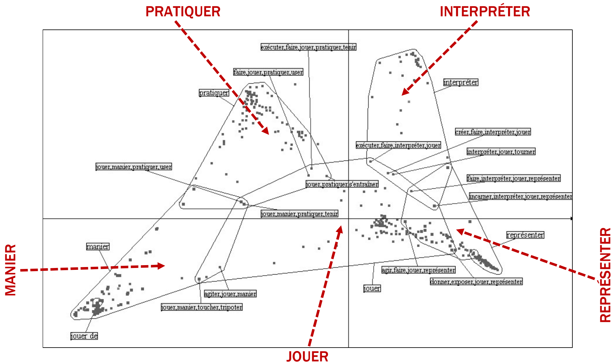
Figure 4 : Visualisation de l'intersection entre la polysémie du v. jouer et de 4 de ses synonymes contextuels { interpréter , manier , pratiquer , représenter } à l'aide du DICTIONNAIRE ÉLECTRONIQUE DES SYNONYMES du CRISCO (cf. François 2005)
