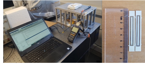
FIGURE 3. a) Photo du banc de mesure utilisé et b) des deux résonateurs utilisés (cuivre sur Rogers RO4003C).
