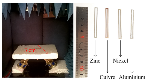
FIGURE 3. a) Installation à l'intérieur de la chambre climatique. b) Résonateurs boucle fabriqués avec différents métaux.
