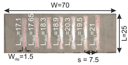
FIGURE 4. Tag fabriqué avec 7 résonateurs et un plan de masse, toutes les dimensions sont en millimètre
