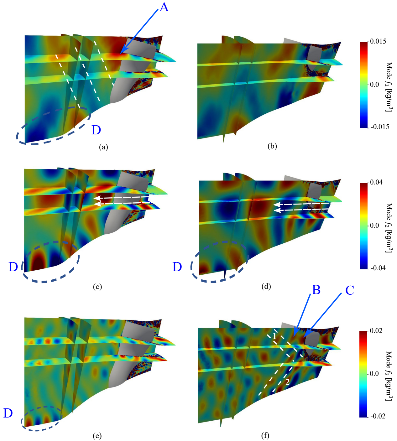
FIG. 23: Spatial distribution of the density modes using the DMT technique. (a) & (b) Mode f_1 . (c) & (d) Mode f_2 . (e) & (f) Mode f_3 .
