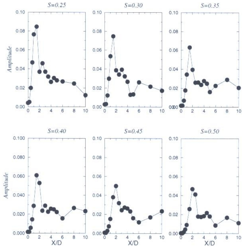
Figure 5: Evolution spatiale du mode global basée sur la composante longitudinale du vecteur vitesse
