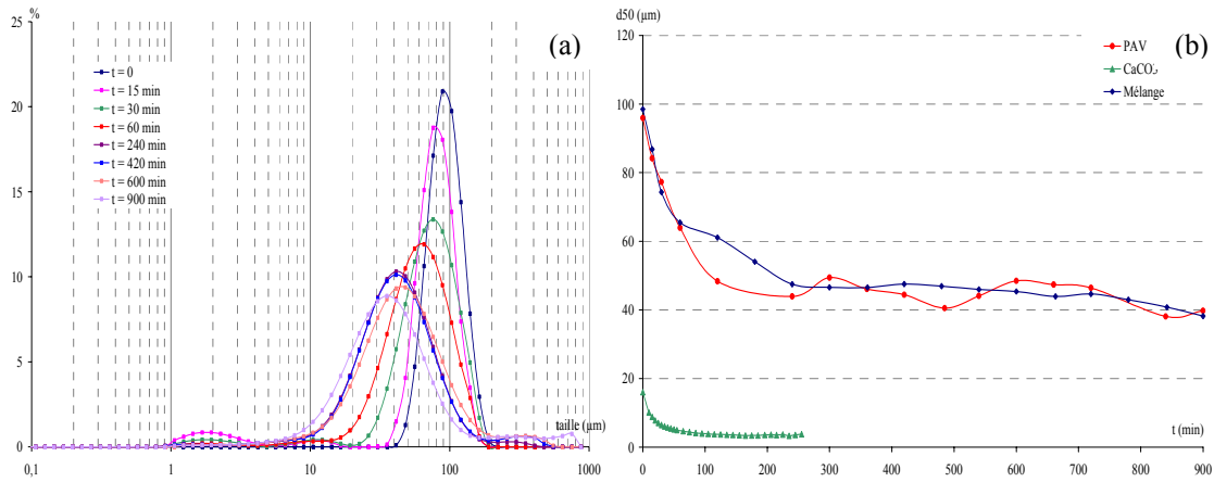
Figure 2. Evolution des distributions granulométriques pour différents temps de broyage du PAV (a). Evolution du diamètre moyen des particules de PAV, carbonate de calcium et du mélange en fonction du temps de broyage (b).
