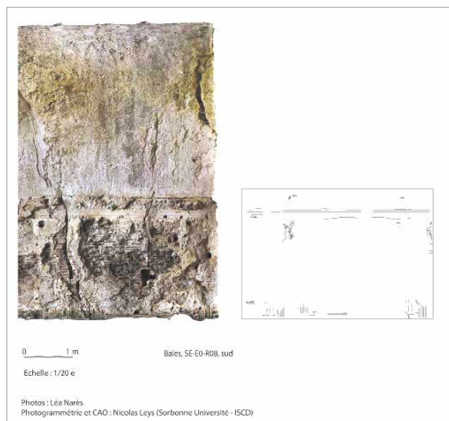
6. Baïes, secteur de Mercure, pièce (c). Photogrammétrie et relevé du mur (© Léa Narès (photos et relevé) et Nicolas Leys (photogrammétrie)).
