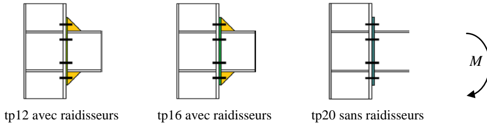
Figure 7. Modèles avec et sans raidisseurs en fonction de t_p .
