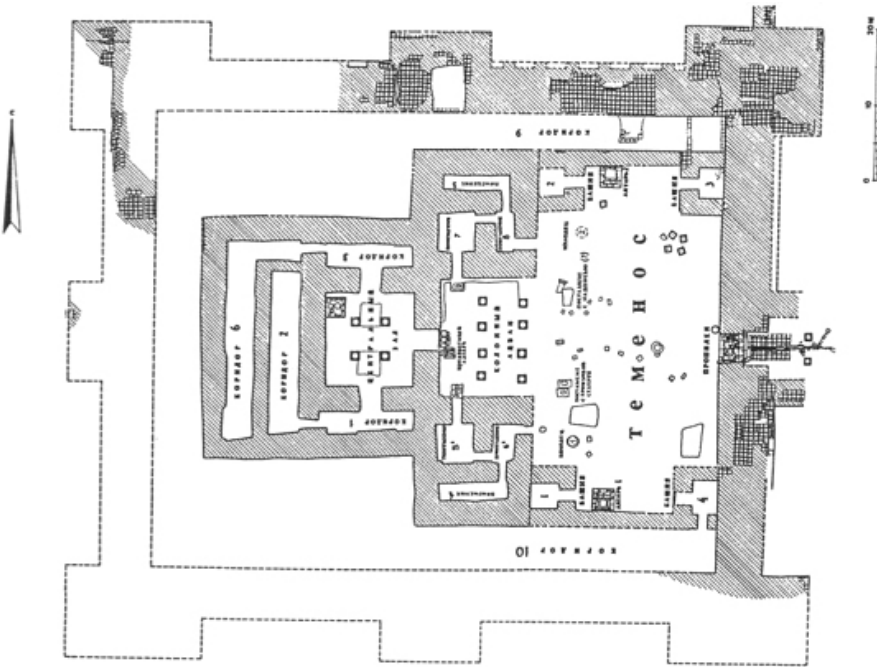
FIG. 4. — Temple de Takht-i Sangin (Tadjikistan), III e siècle av. n. è., plan (G. Lindström, S. Hansen, A. Wiczorek et M. Tellenbach éd., Zwischen Ost und West. Neue Forschungen zum antiken Zentralasien , fig. 4).
