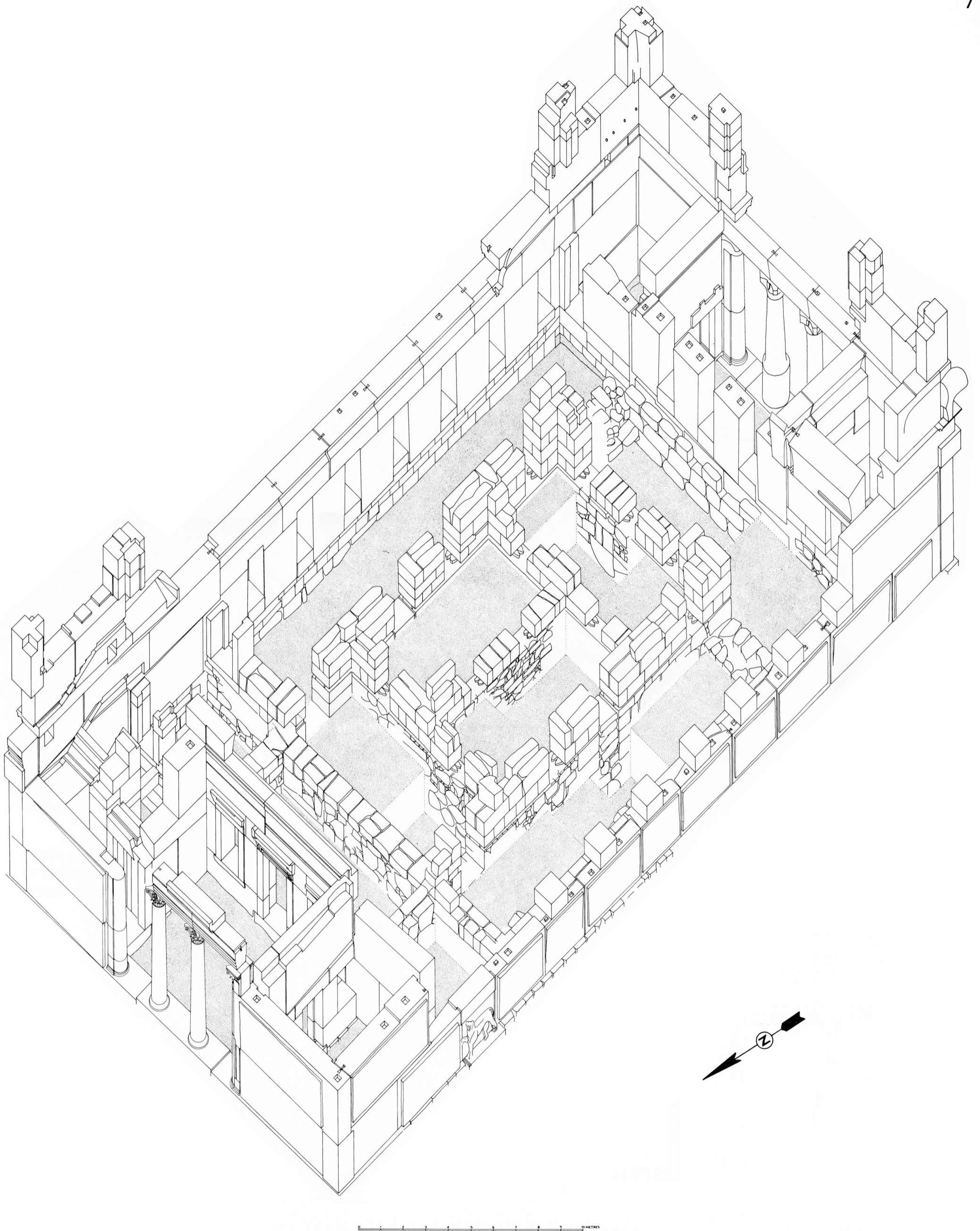
7. Vue axonométrique du Qasr au niveau 1 restitué.
