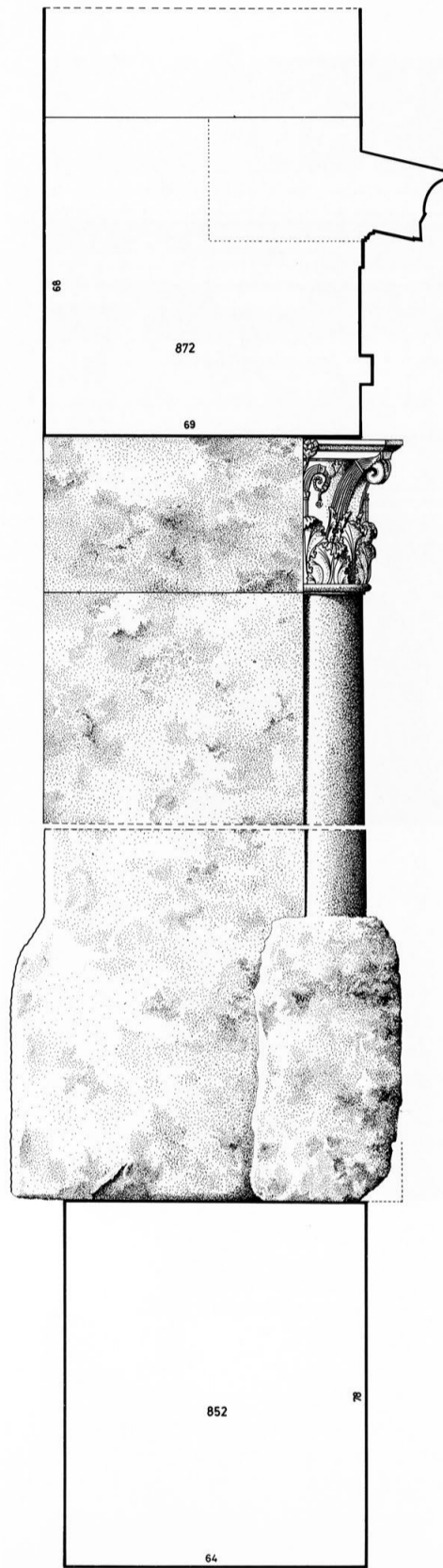
COUPE DU MUR 8
