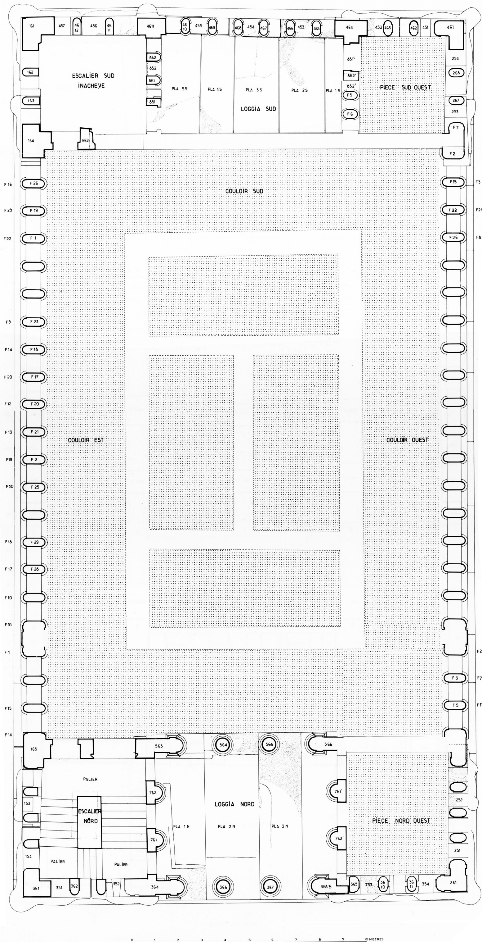
10. Plan restitué du niveau 2.
