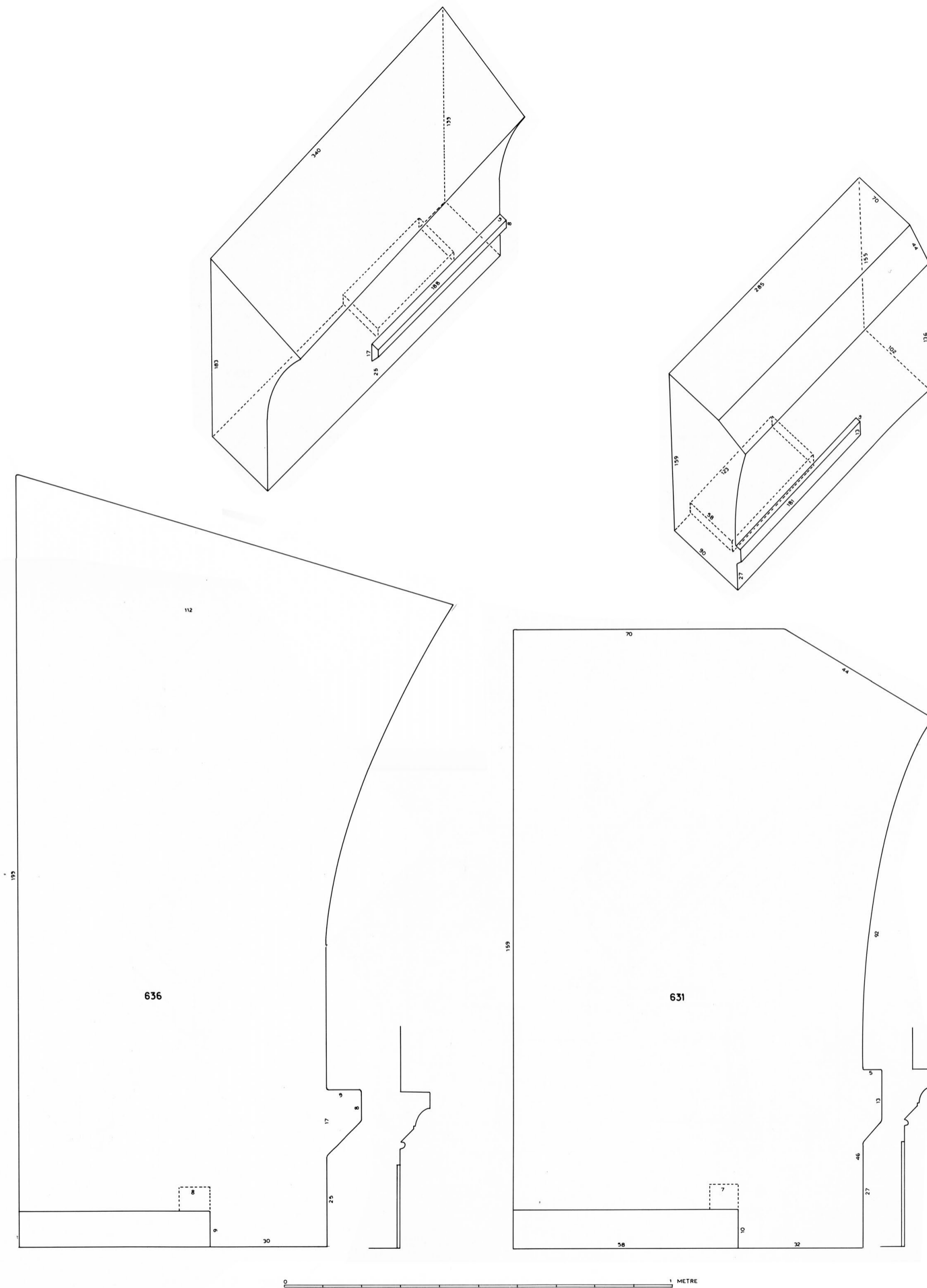
88. Linteaux: pièce sud-ouest (bloc 636) et cage d'escalier sud (bloc 631).
