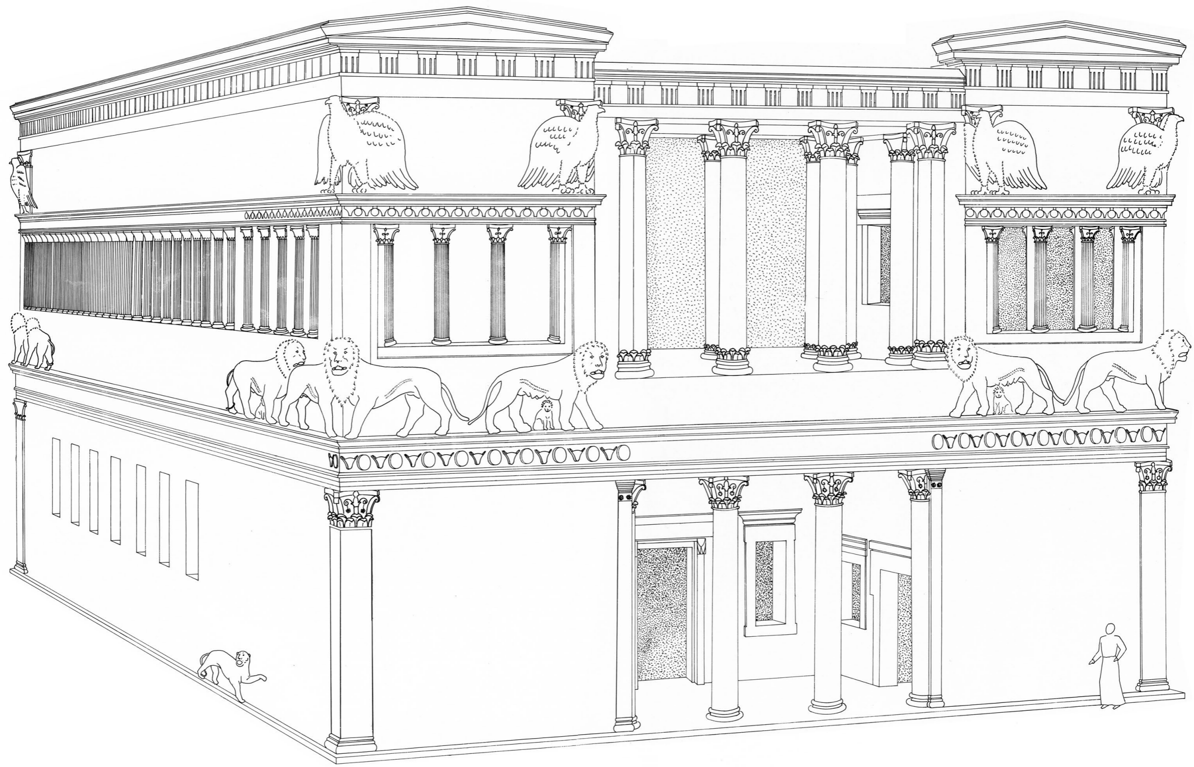
100. Iraq al Amir, Qasr el 'Abd: vue perspective restituée.
