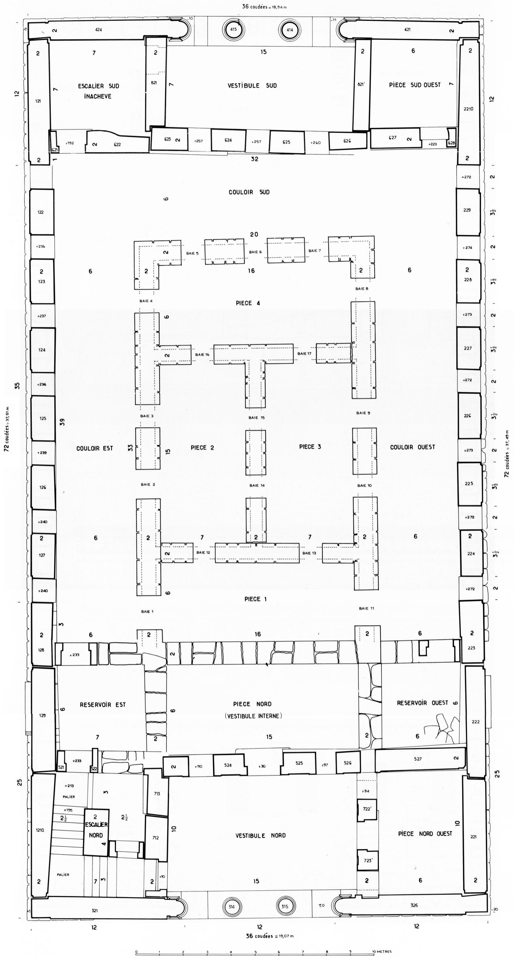
9. Plan restitué du niveau 1 à la cote 2.80 (mesures en coudées).
