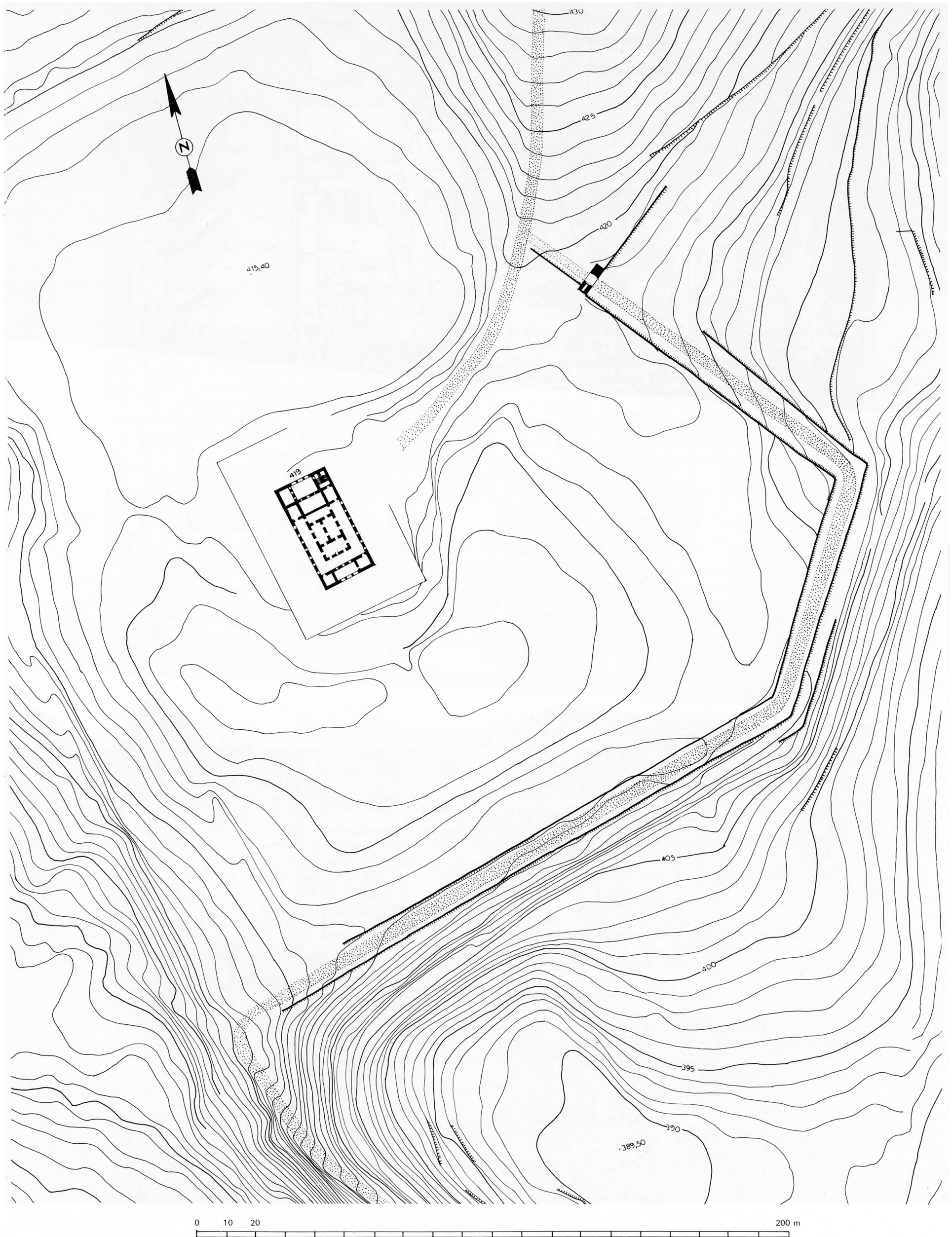
3. Le Qasr al 'Abd: la digue, le lac et la porte du domaine (état antique restitué).
