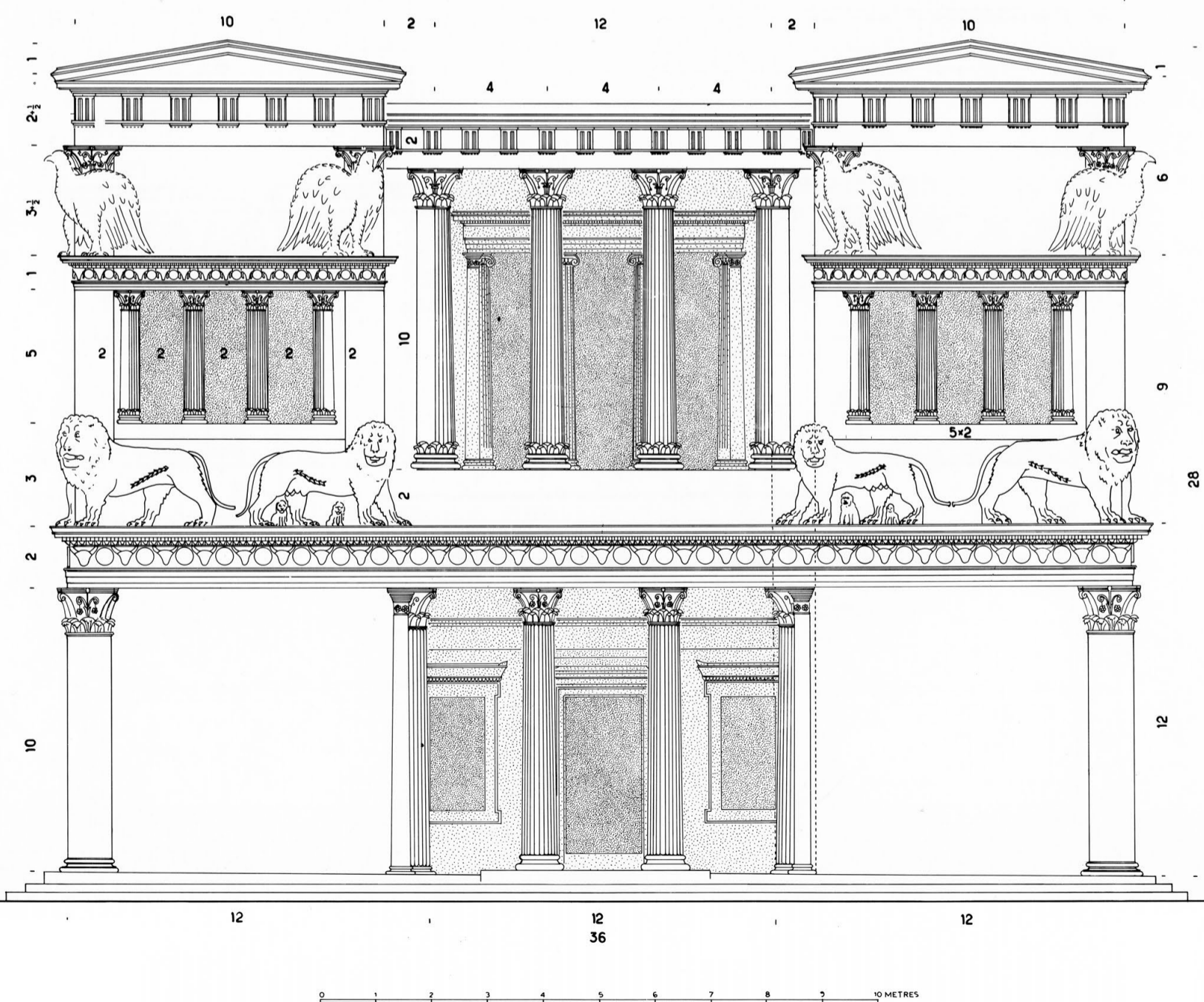
36. Coupe restituée sur le vestibule nord. — Façade nord restituée (mesures en coudées).
