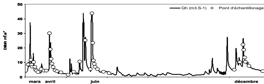
Figure 2. Variations des débits horaires de la Save à Larra au cours de la période d'étude (mars à décembre 2008)
