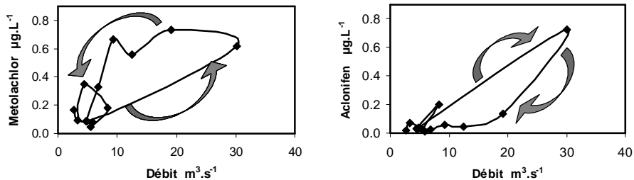
Figure 4. Relations entre les concentrations en métolachlore (à gauche) ou acлонifen (à droite) et les débits au cours de la crue d'avril 2008 sur la Save à Larra. Phénomènes hystérésis entre montée et descente de crue
