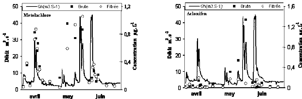
Figure 3. Variations des débits et des teneurs en métolachlore (à gauche) et Aclonifen (à droite) dans l'eau brute (carré noir) et l'eau filtrée (rond blanc) au cours des crues d'avril et de juin 2008 sur la Save à Larra
