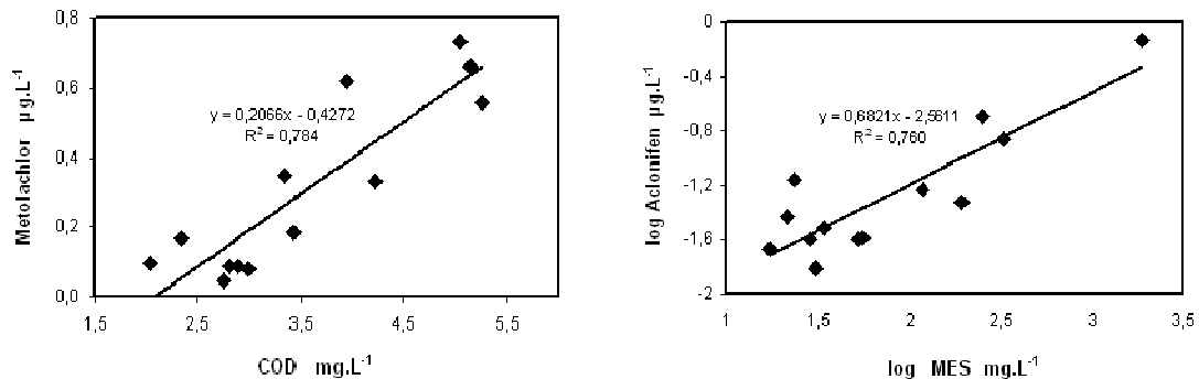
Figure 5. Relations entre les teneurs en métolachlore et en COD (à gauche) et entre les teneurs en acлонifen et MES (à droite) au cours de la crue d'avril 2008 sur la Save à Larra
